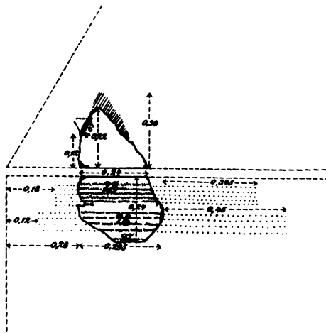
fig. X (1:20).
